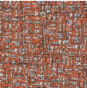
QRC118-190 SYNTAX
