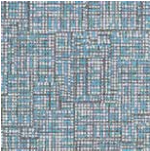
DAT104-153 XML
