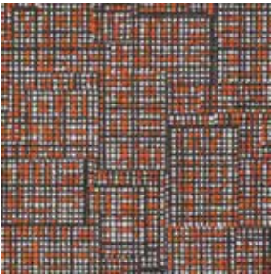
DAT190-118 SYNTAX
